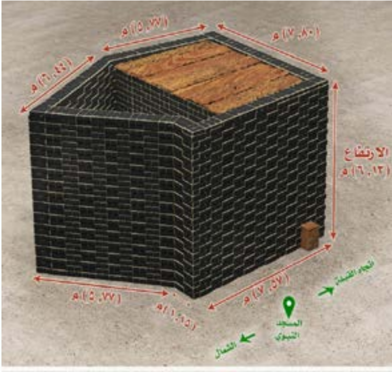
(Beşgen ve kare duvarın temsili çizimi)
